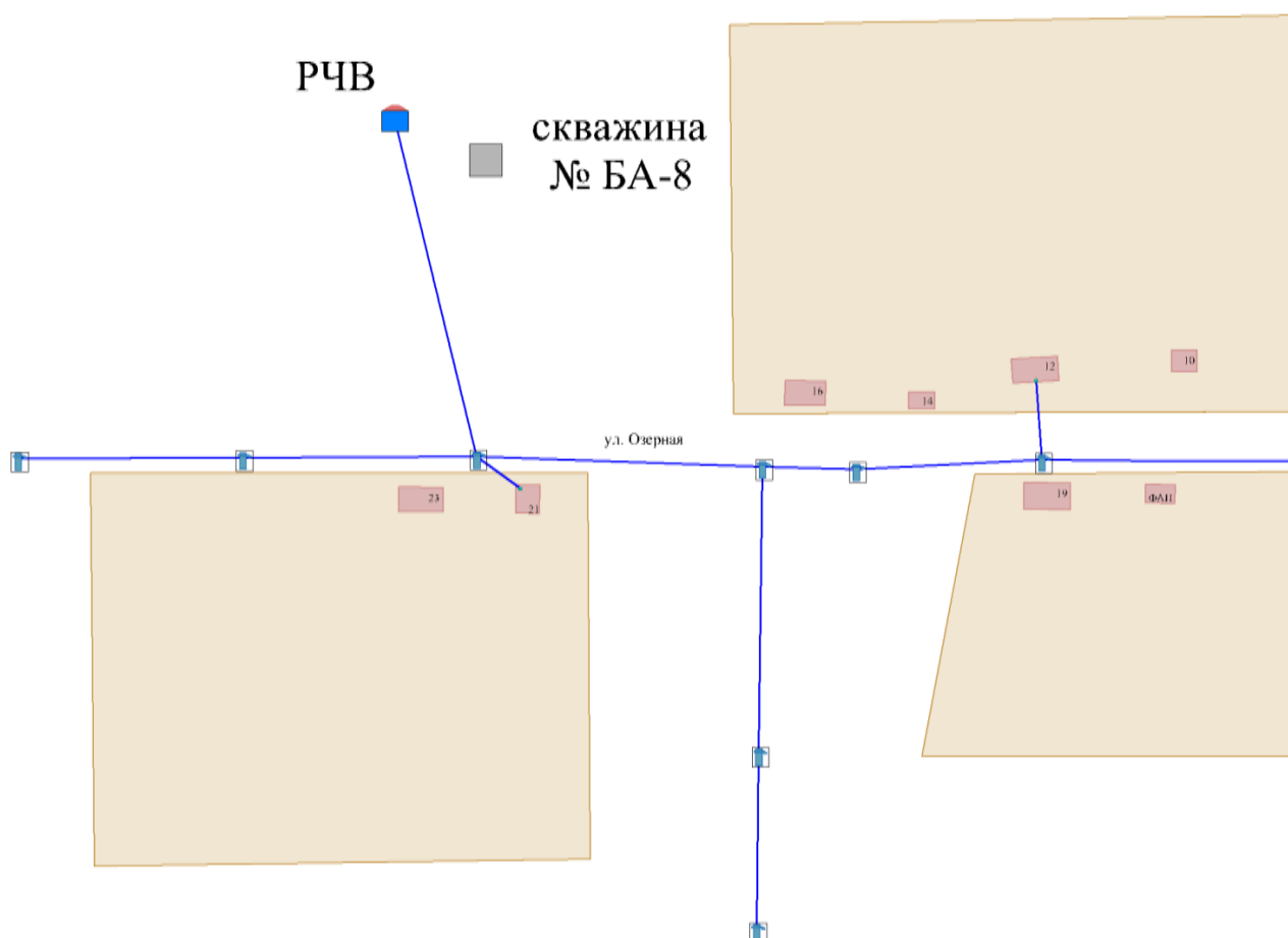
Рисунок 6.2 – Схема существующего размещения объектов централизованной системы водоснабжения
