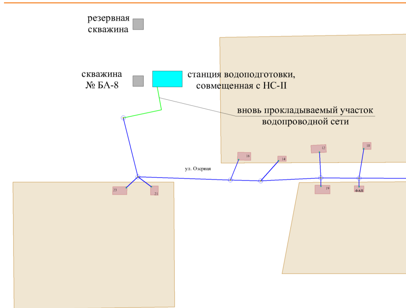
Рисунок 6.3 – Схема планируемого размещения объектов централизованной системы водоснабжения
